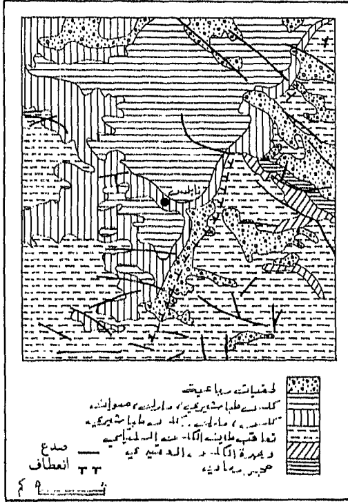
( عن الخارطة الجيولوجية للاردن ، مقياس ١ : ٢٥٠,٠٠٠ )
